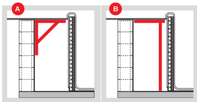
Varianta s nosnými úhelníkovými profily (doporučujeme)
