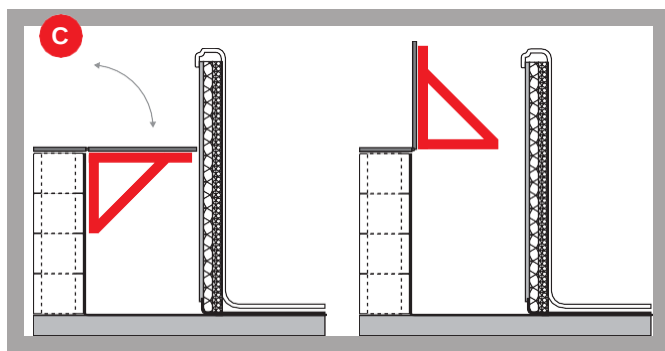
Varianta s úhelníkovými profily na ocelových pantech (ideální pro polozapuštěné varianty)
